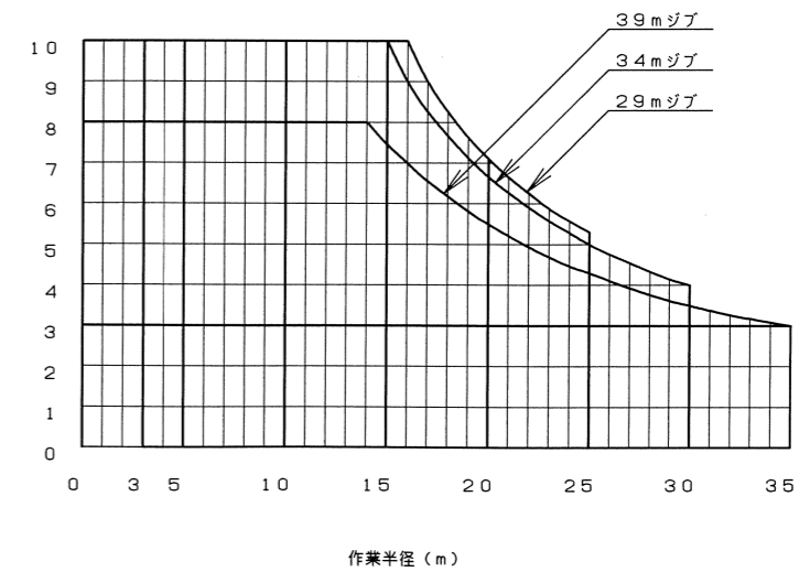
定格荷重線図
